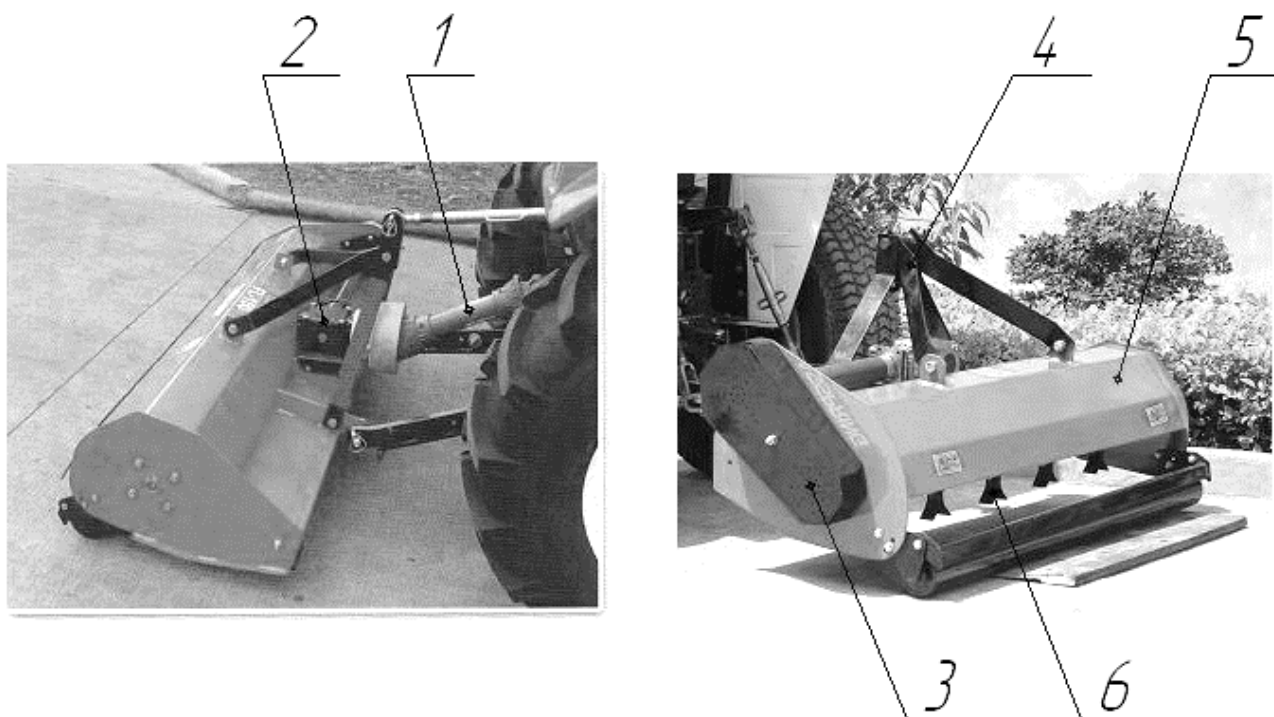
Рис.1 Устройство косилки
