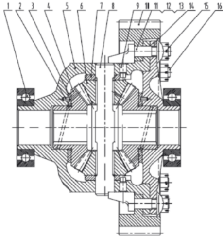
Рис. 3.10а. Дифференциал (3x2+1) в сборе.
