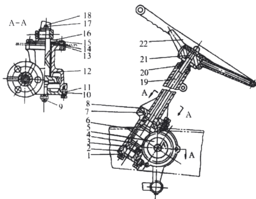
Рис. 3.14. Рулевое управление.
