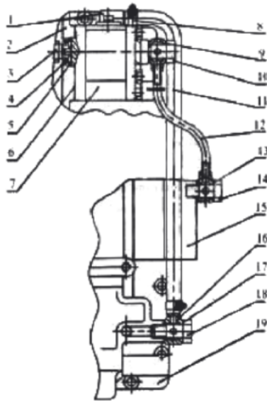
Рис. 3.33. Гидравлическая система.
