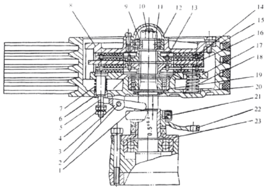
Рис. 3.2. Сцепление.
