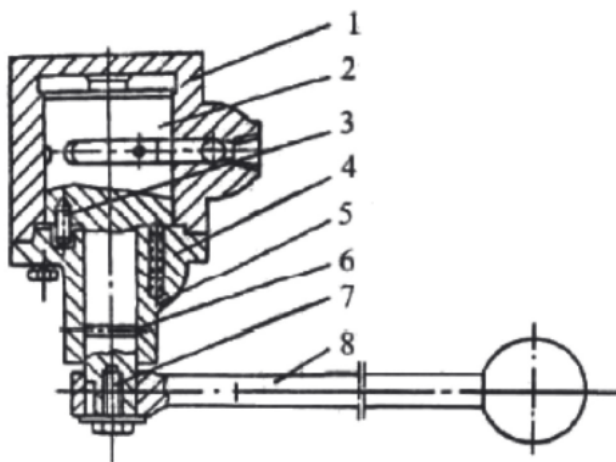
Рис. 3.28. Контрольный клапан.
