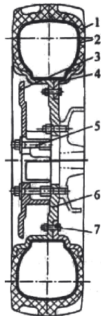
Рис. 3.25. Заднее колесо со сборным ободом обода.
