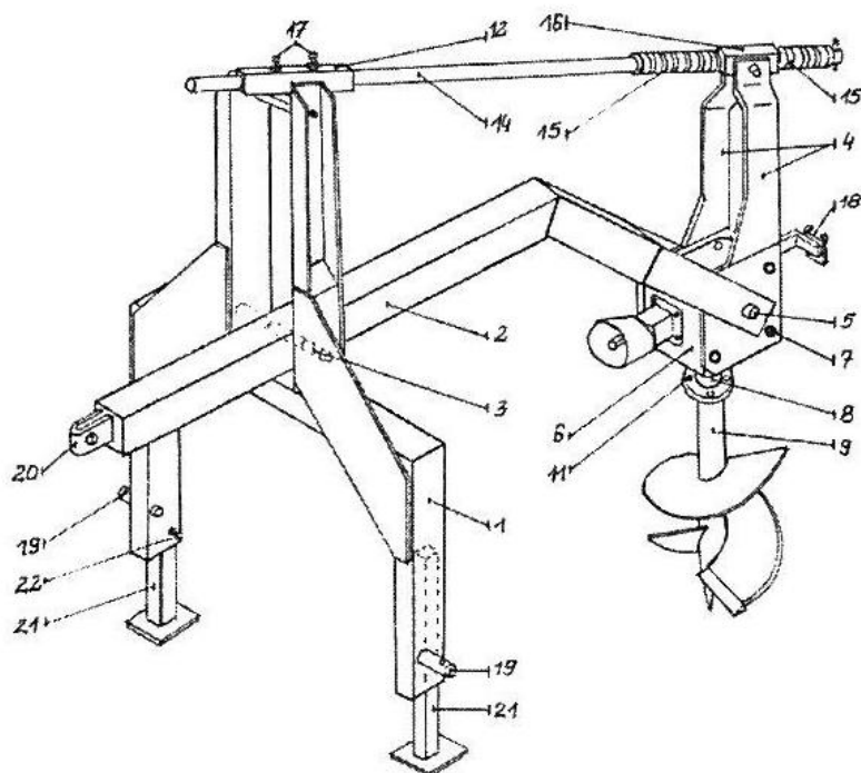
Рис. 1 Составные элементы, земляного бура
