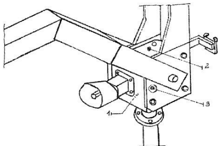
Рис. 2. Места замены и контроля масла в передаче
