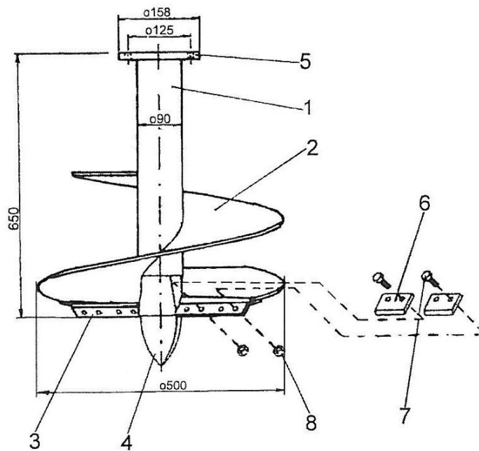
Рис. 4А Бур Ø 50 см, длина 65 см
