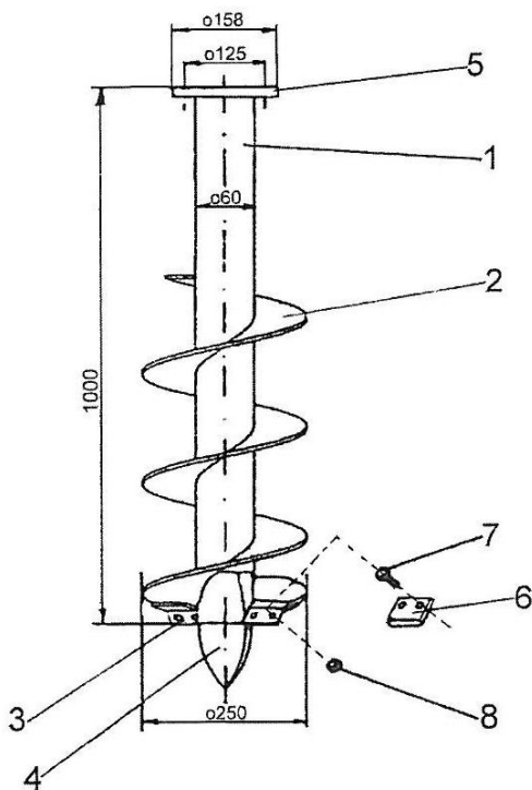
Рис. 4 Бур Ø 25 см, длина 100 см
